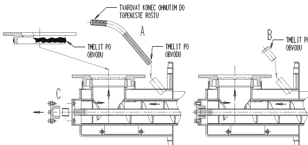
Obrázek č. 1.3 (Hořák ROJEK 25)
