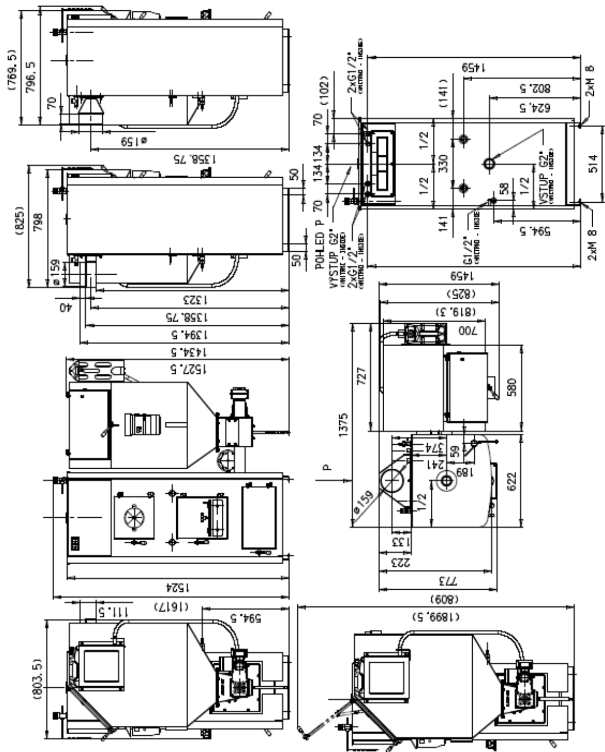
Obrázek č. 5.5 (TKA 15 s 300 l nekapotovanou násypkou)
