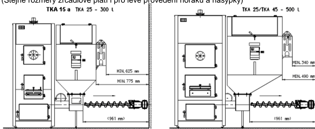
Obrázek č. 8 (Vysunutí šneku – informativní obrázek)
