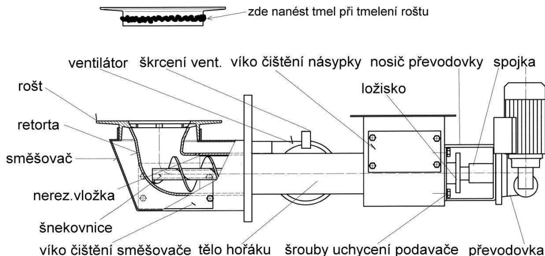
Obrázek č. 1 (Hořák ROJEK 15)
