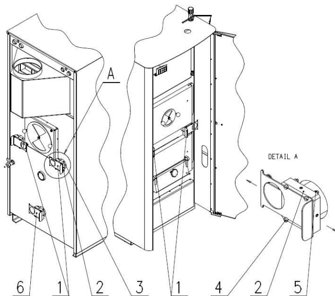
Obrázek č. 15 (Informativní TKA 45)
