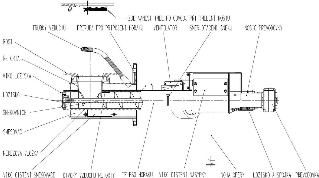
Obrázek č. 1.1 (Hořák ROJEK 25)
